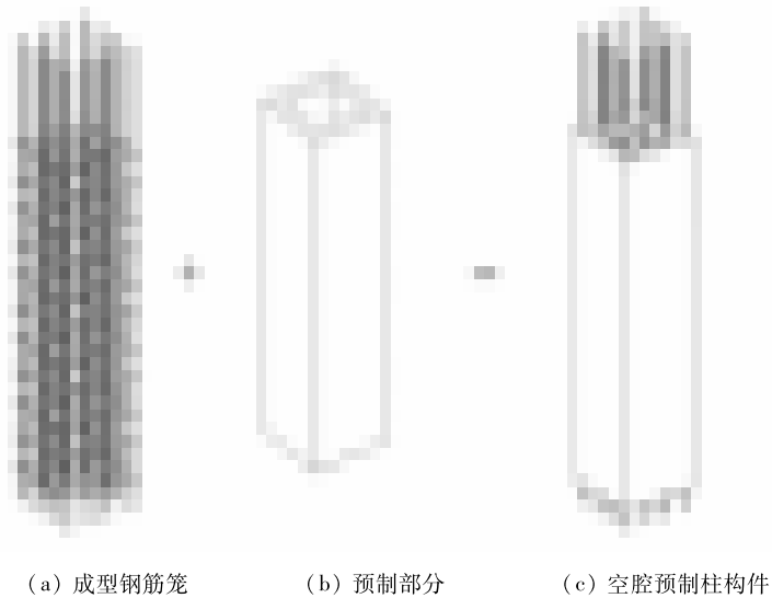
图3 空腔预制柱构件三维图
