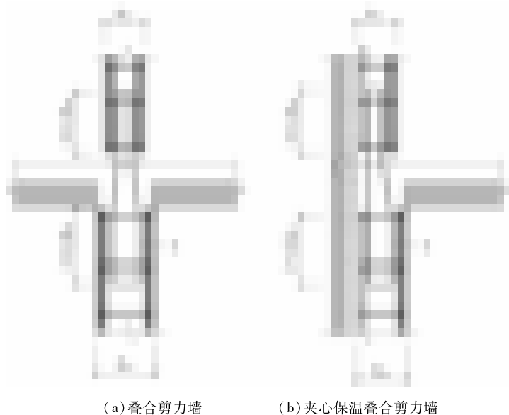
1—弯折环状连接筋; b_{w1} —下层叠合剪力墙厚度; b_{w2} —上层叠合剪力墙厚度
