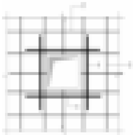
1—洞口补强钢筋;2—墙体钢筋
