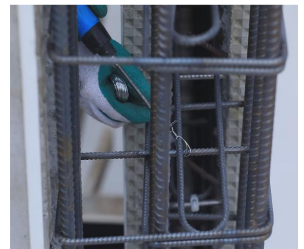
环筋绑扎
