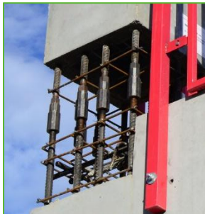
可调组合直螺纹套筒连接
