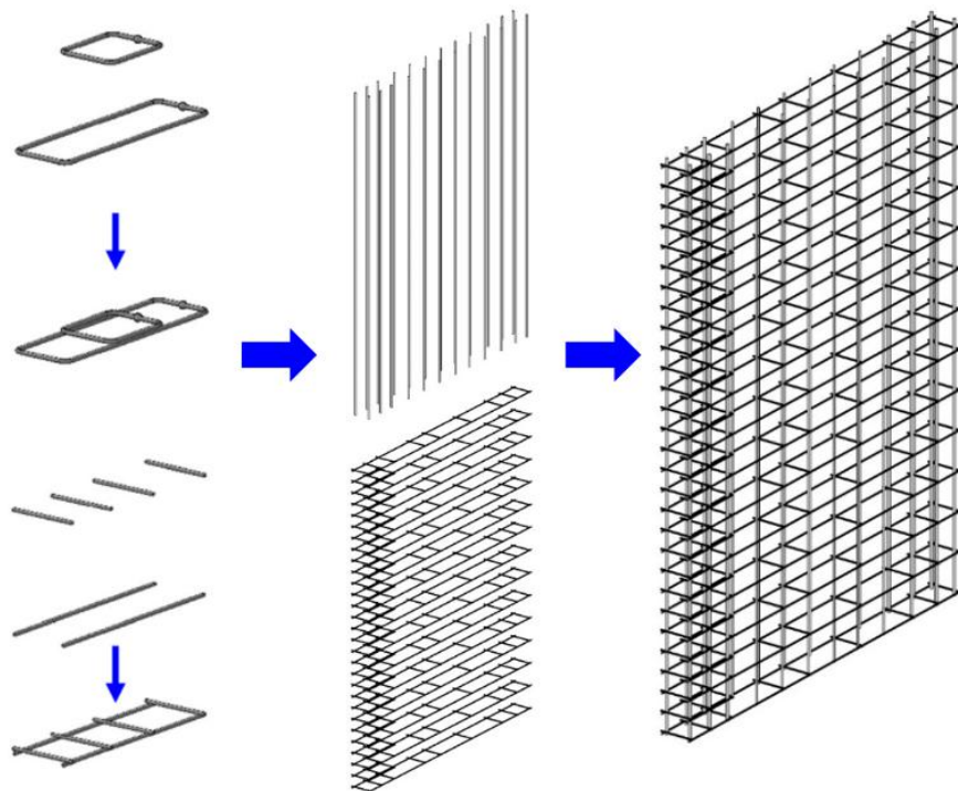
① 焊接钢筋网片 ② 钢筋网片与纵筋焊接 ③ 钢筋笼
