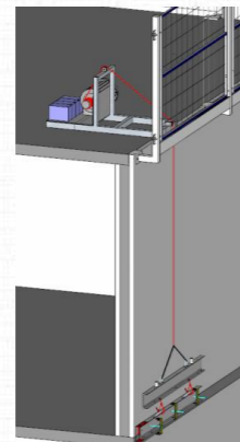
浇筑混凝土后通过定制的电动或手动工具拆除
