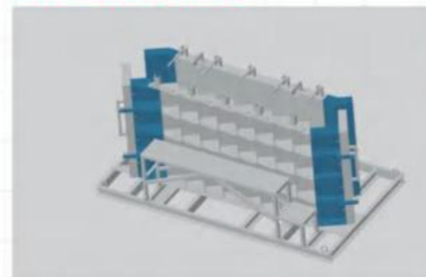
• 组合式楼梯模具
