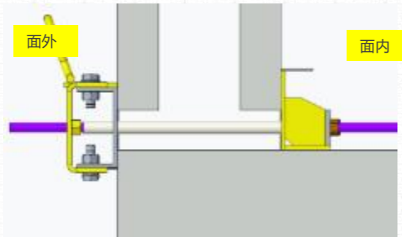
底部封堵节点模板构造
