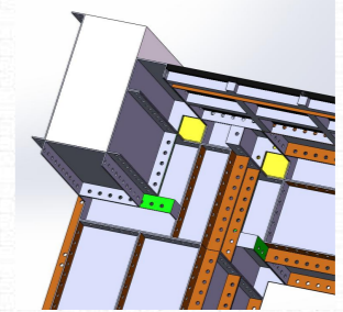
骨架+面板安装细部大样
