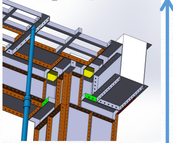
骨架安装细部大样
