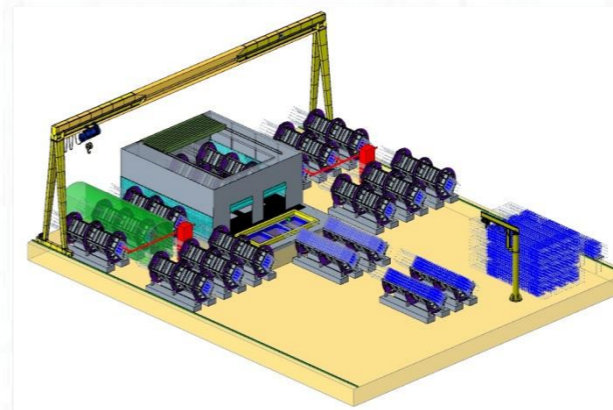
空腔柱生产线布局
