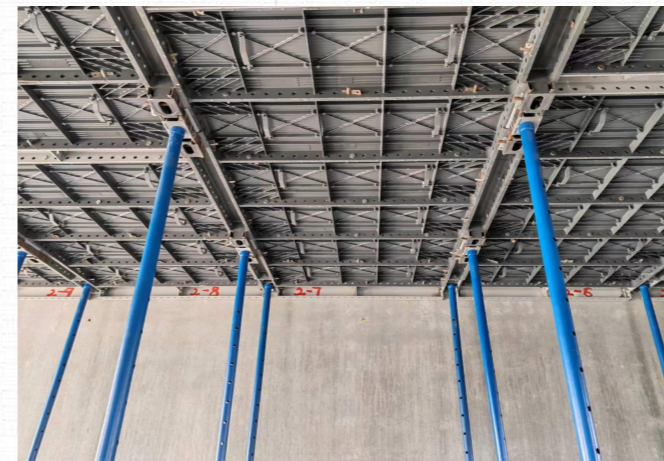
● 铝/镁合金楼面模板
