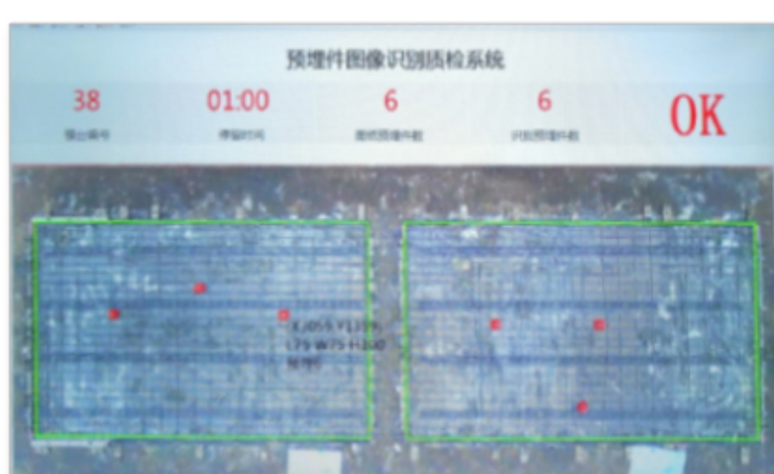
视觉预埋安装自动质检
