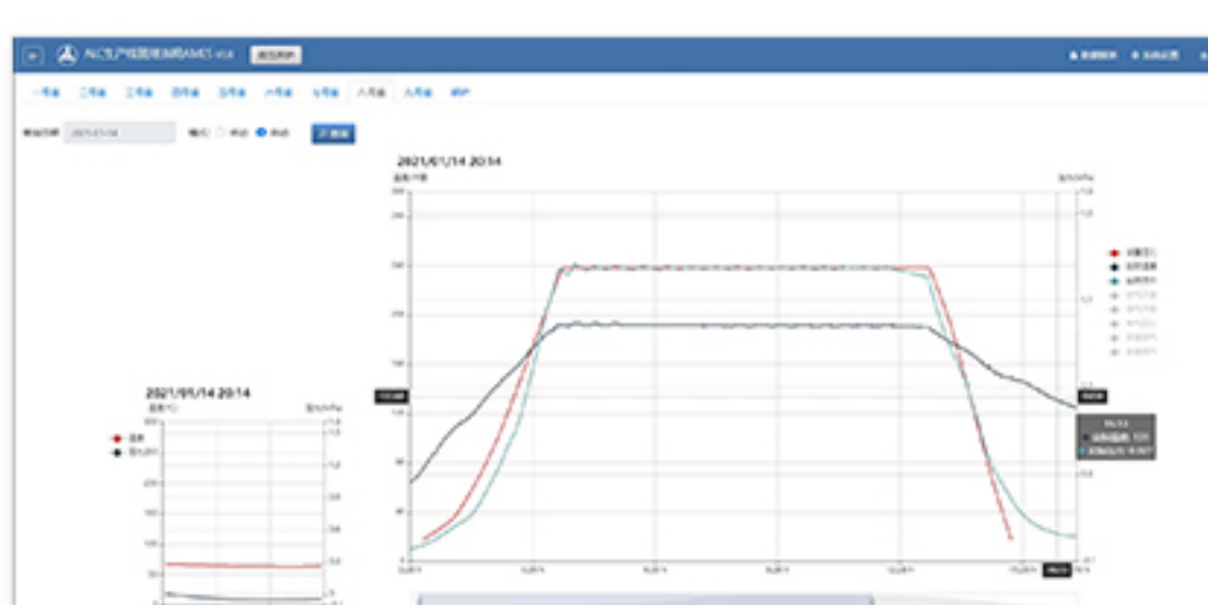
蒸养工艺曲线
