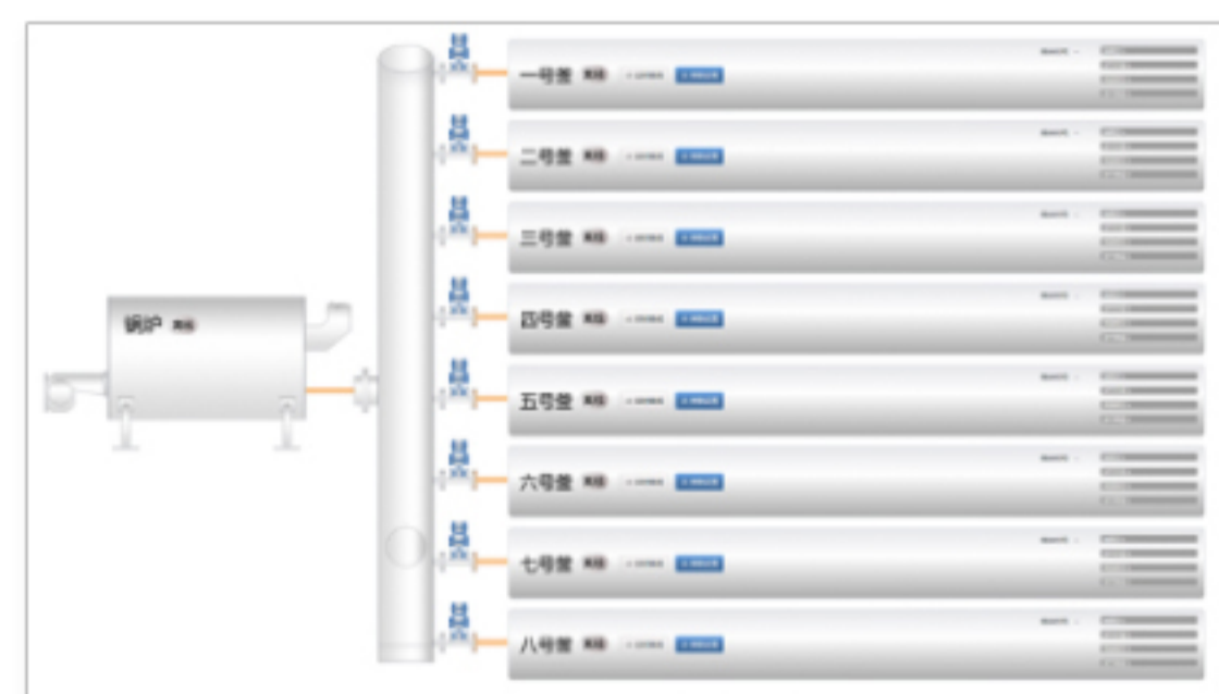
自动蒸养
