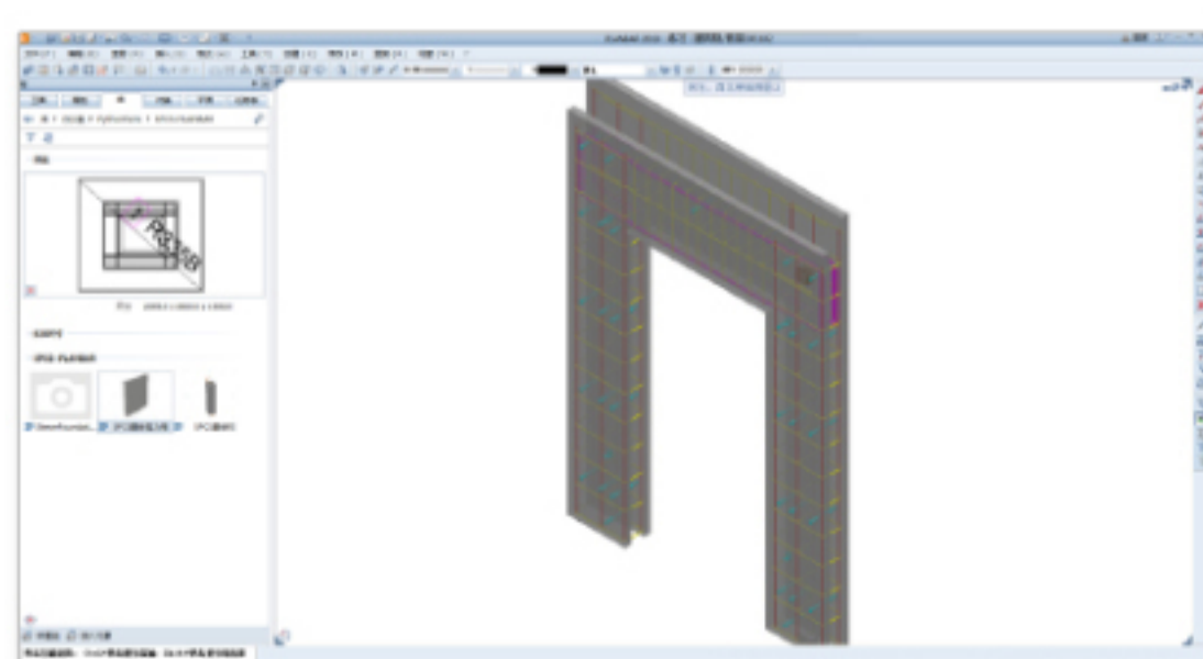
SPCS墙设计
